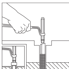
Ringschlüssel aufschieben und herausdrehen.
